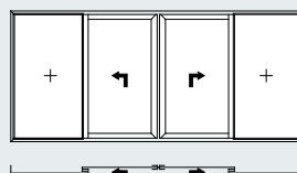
Tipo 1D.i Scorrevole internamente
